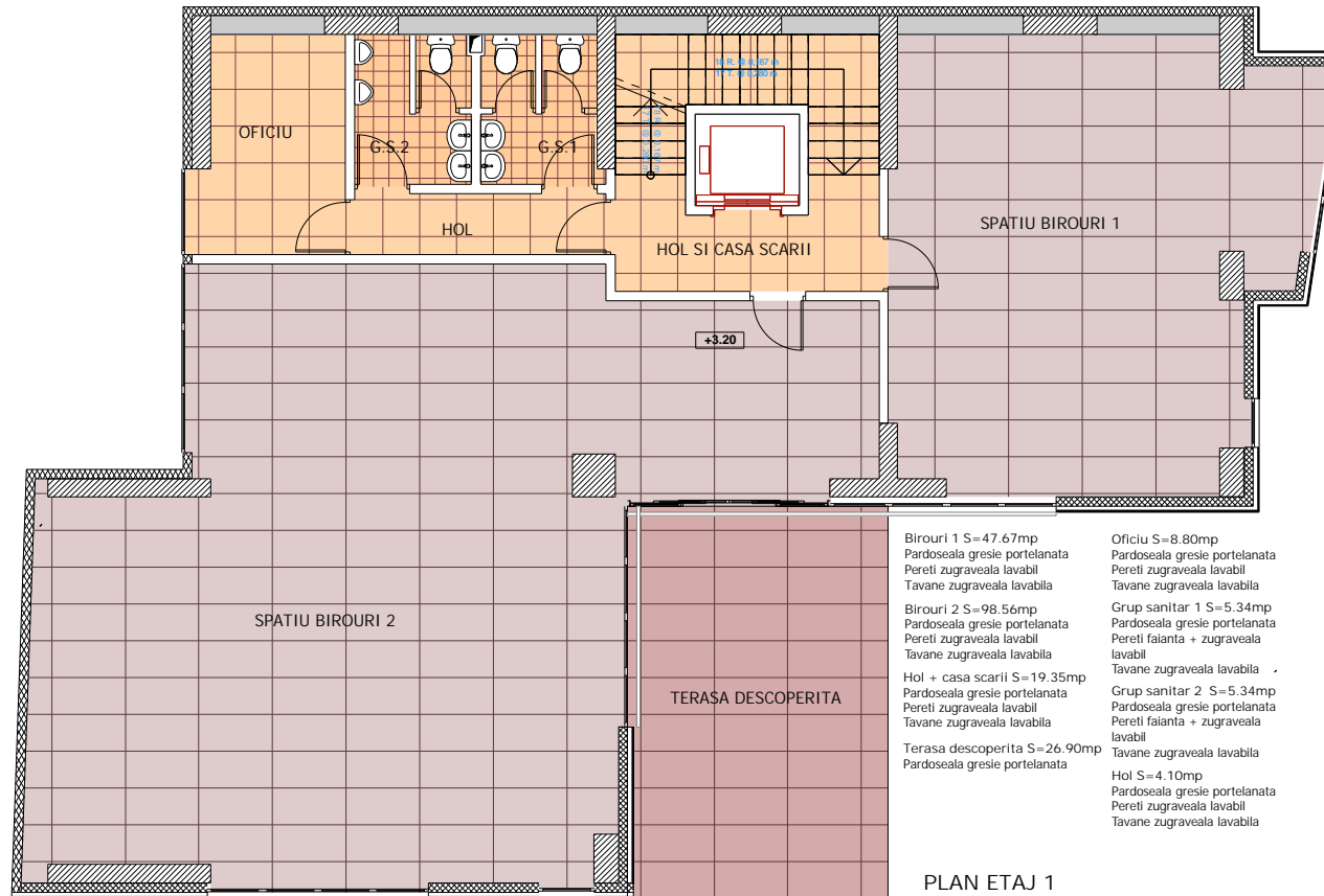
PLAN ETAJ 1
